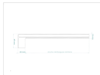
Tapa lateral izquierda Remate de aluminio para el extremo izquierdo
