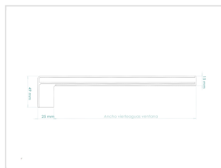
Tapa lateral esquerra Remat d'alumini per a l'extrem esquerre
