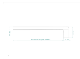
Tapa lateral dreta Remat d'alumini per a l'extrem dret
