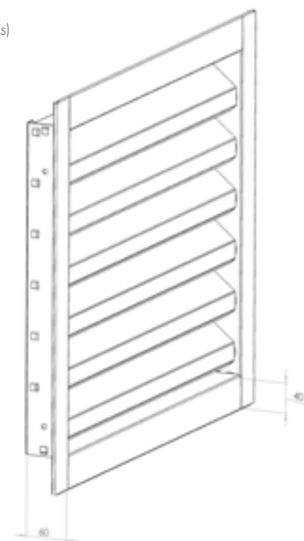
Rejilla antipájaros
