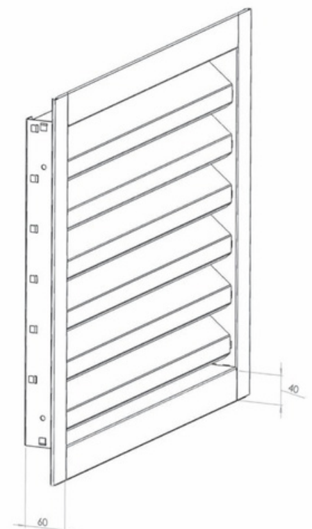
Vogelschutzgitter
